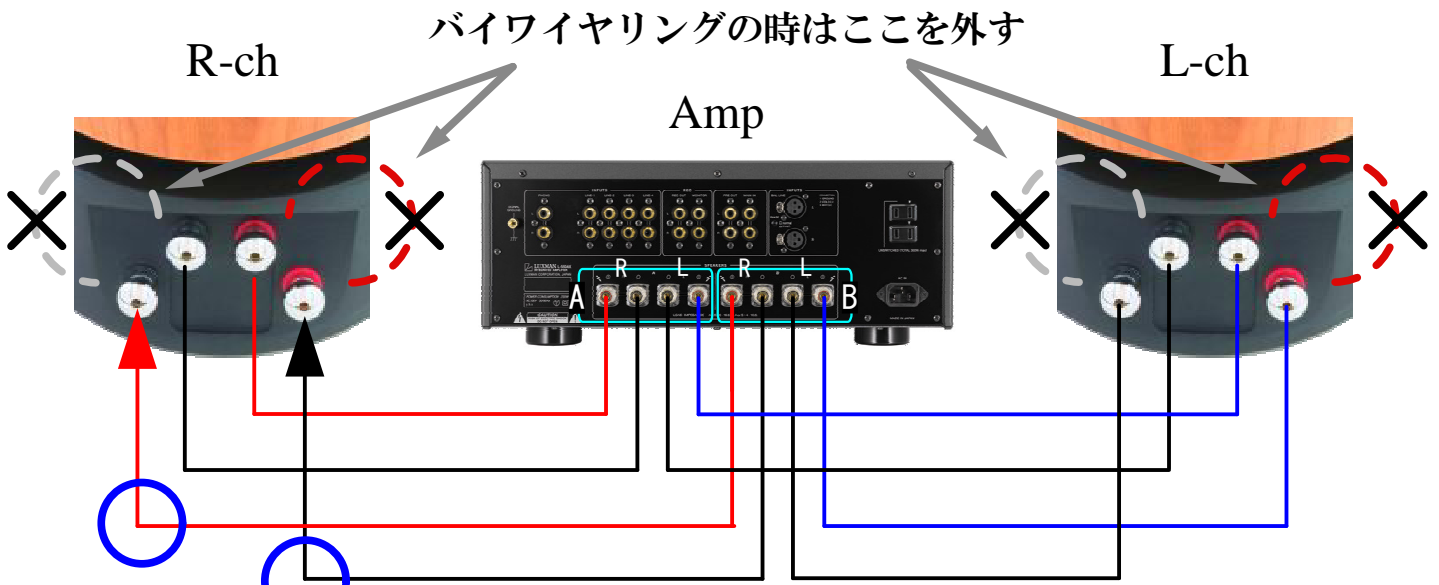
[図1] シングルアンプのバイワイヤリング接続
