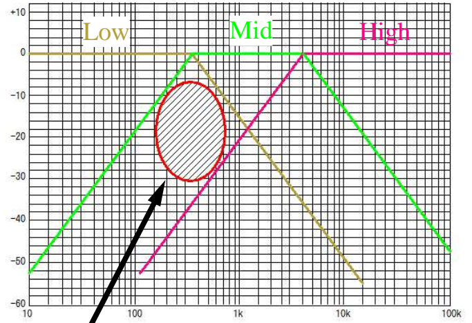
[図3] L/C Networkの特性
