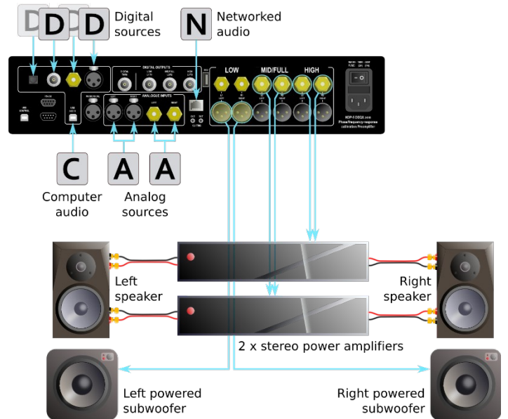
[ バイアンプスピーカー + ステレオサブウーファの接続例 ]
